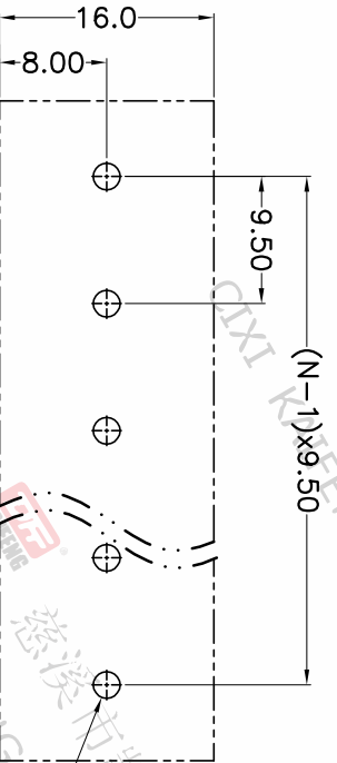
P.C.B. LAYOUT
